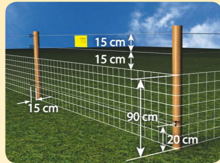
Rys. 3. Fragment ogrodzenia siatkowo-elektrycznego.
