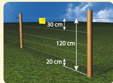
Rys. 2. Fragment stacjonarnego ogrodzenia elektrycznego.
