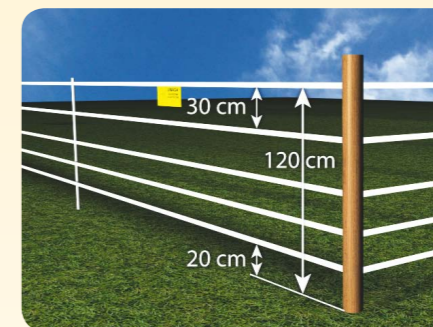
Rys. 1. Fragment przenośnego ogrodzenia elektrycznego.
